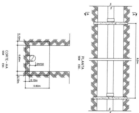
DETALHE DOS BLOCOS DE ANCORAGEM PARA TRECHOS COM DECLIVIDADE > A 20%
