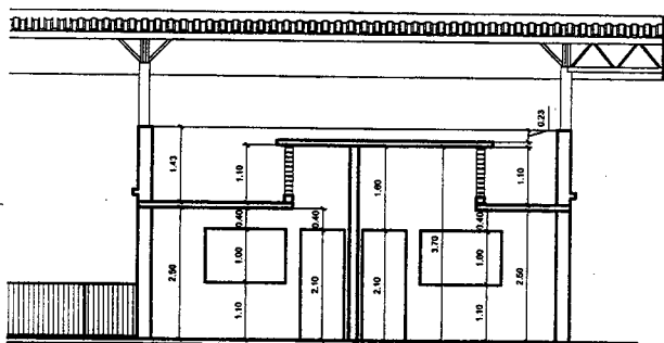
3 CORTE - BB 2/2 ESCALA: 1:75
