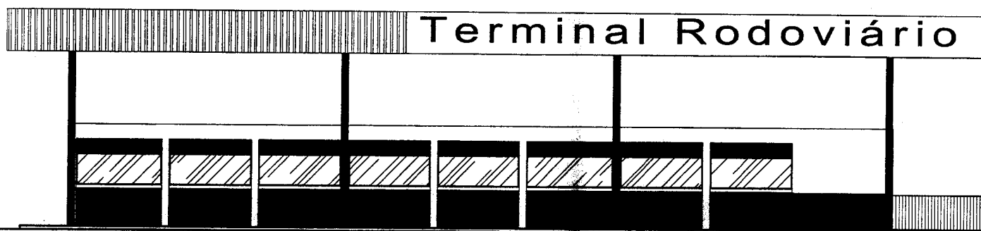
5 FACHADA 2/2 ESCALA: 1:75
